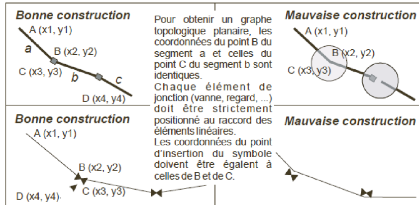
Construction graphique
